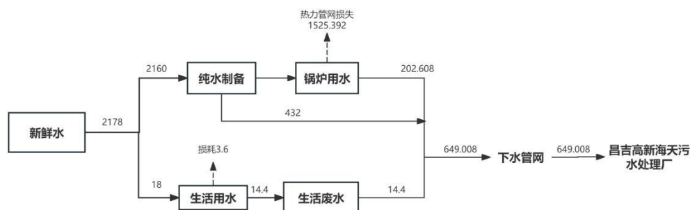
图2-1 项目水平衡 (m 3 /a)
