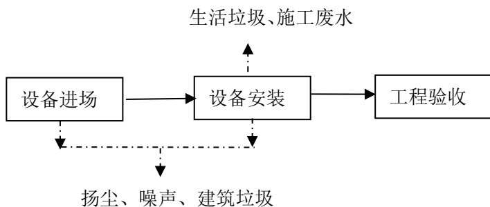
图 2-3 主体工程工艺流程及产污环节图
