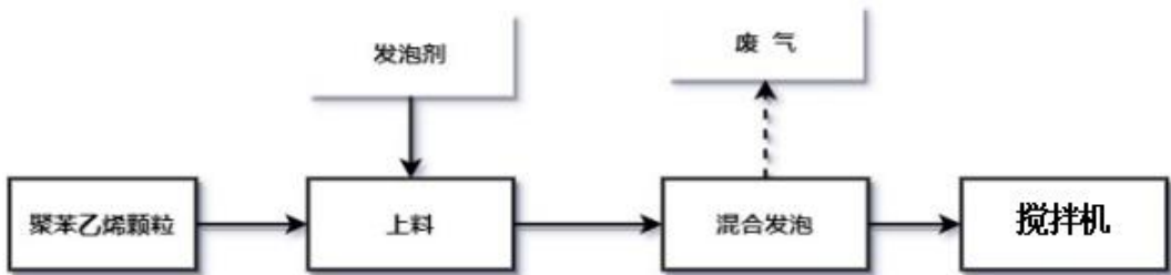
图 2-4 聚苯乙烯发泡生产工艺及产污节点图
