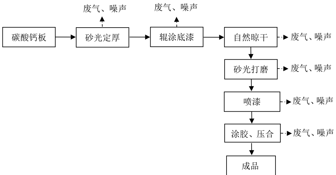
图 2-6 保温装饰一体板生产工艺流程及产污节点图
