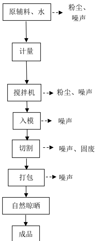
图 2-4 自保温砌块生产工艺流程及产污节点图
