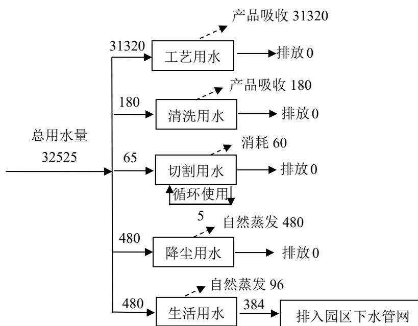
图 2-2 项目水平衡图 (m³/a)
