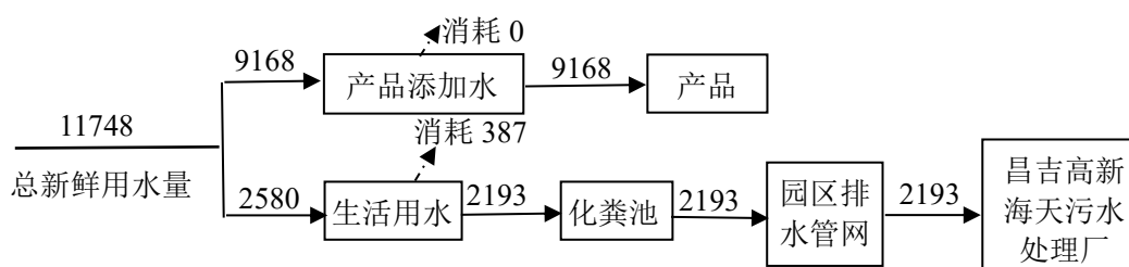
图 2-1 项目水平衡图（m 3 /a）
