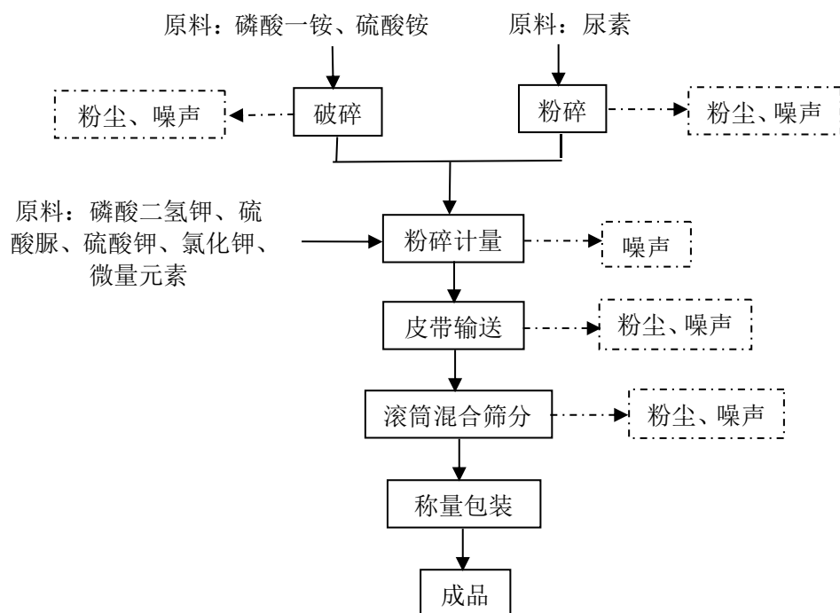
图 2-4 20-25 吨/小时水溶性肥科（固体）生产线生产工艺流程及产污环节图
