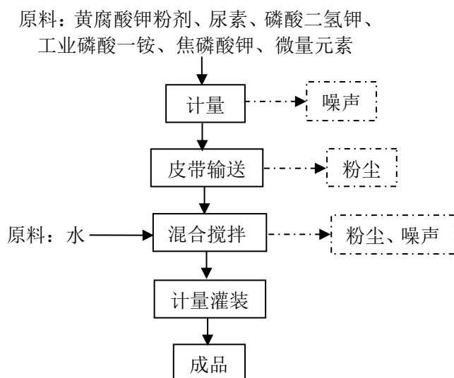
图 2-5 5-25 公斤水溶肥（液体）灌装生产线生产工艺流程及产污环节图
