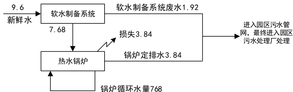
图 2-1 项目水平衡图 \text{m}^3/\text{d}
