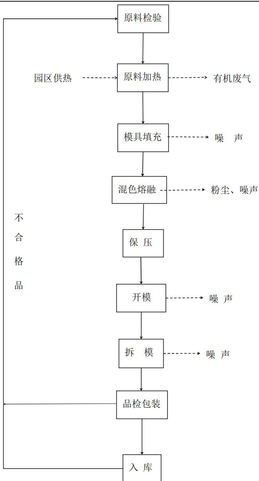
图 2-4 现有工程工艺流程及产排污节点图
