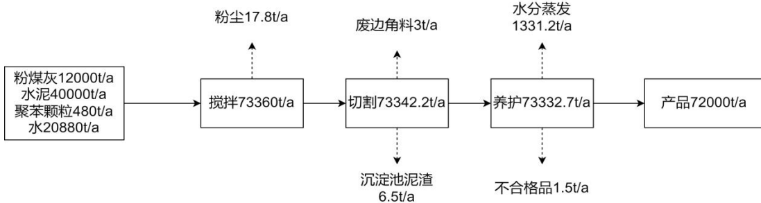
图 2-1 项目物料平衡图
