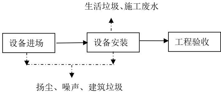
图 2-3 主体工程工艺流程及产污环节图
