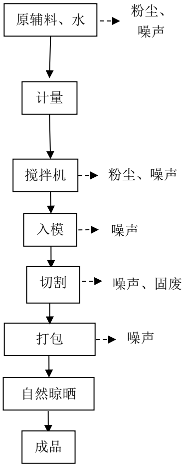
图 2-4 匀质自保温砌块生产工艺流程及产污节点图
